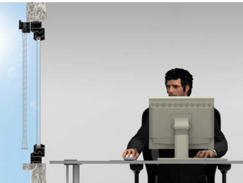
Abb. 7 Cut Off Stellung der Lamellen. Die Lamellen werden so geneigt, dass die Sonneneinstrahlung abgeschirmt, aber die Sichtverbindung nach außen und Tageslichteinfall noch möglich ist.
