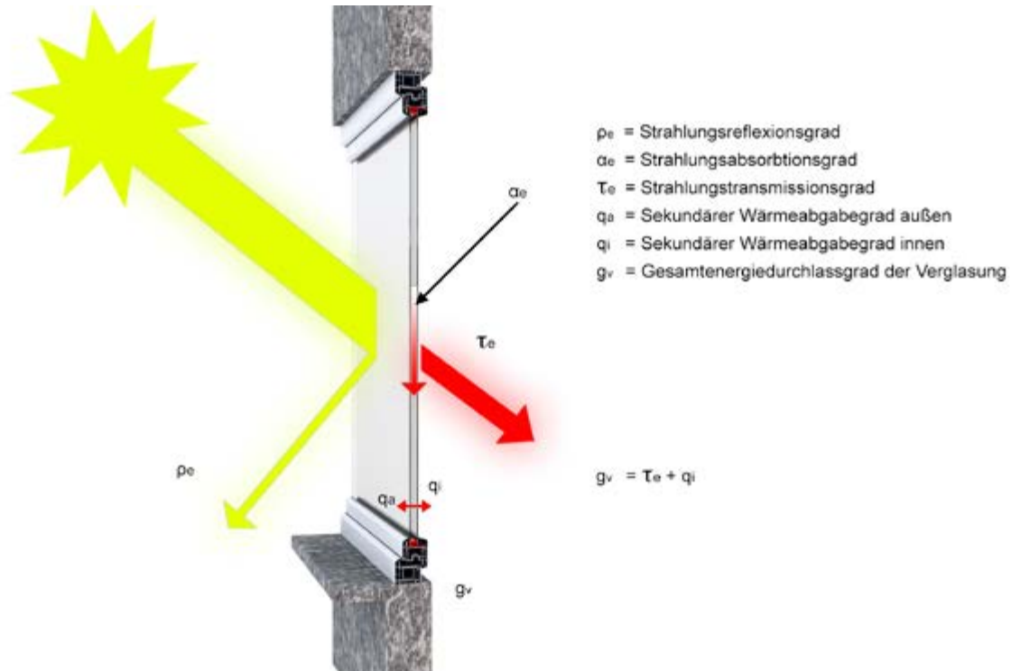
Abb. 3 Transmission, Reflexion, Absorption an einer Wärmeschutzverglasung
